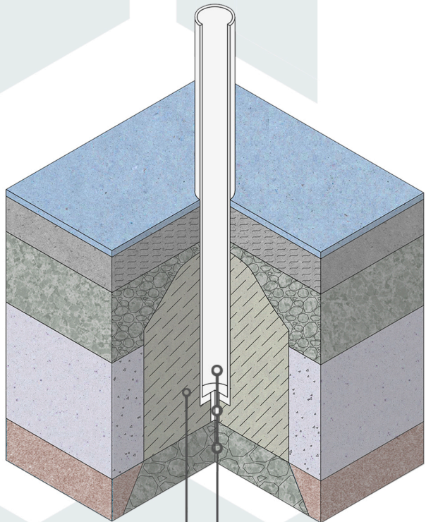
СХЕМА МОНТАЖА СТОЙКИ МАФ
