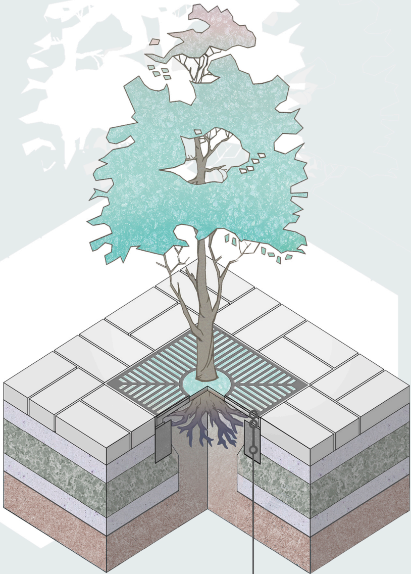
СХЕМА УСТРОЙСТВА ЗАЩИТЫ КОРНЕЙ ОТ ВЫТАПТЫВАНИЯ
